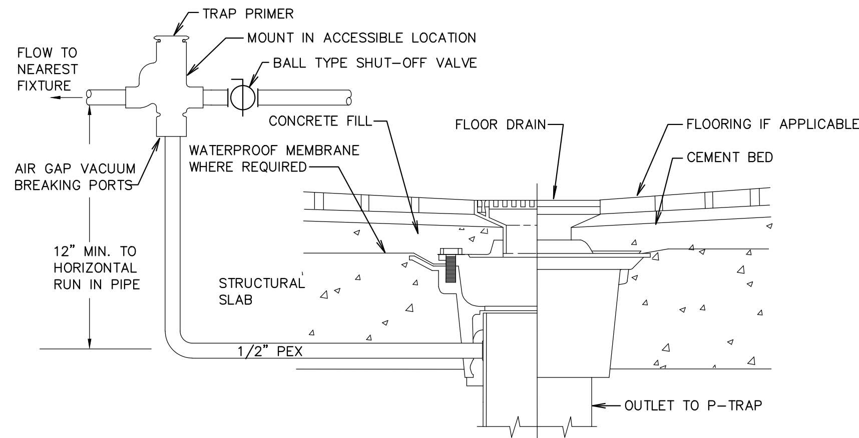
F TRAP PRIMER DETAIL SCALE: NONE
