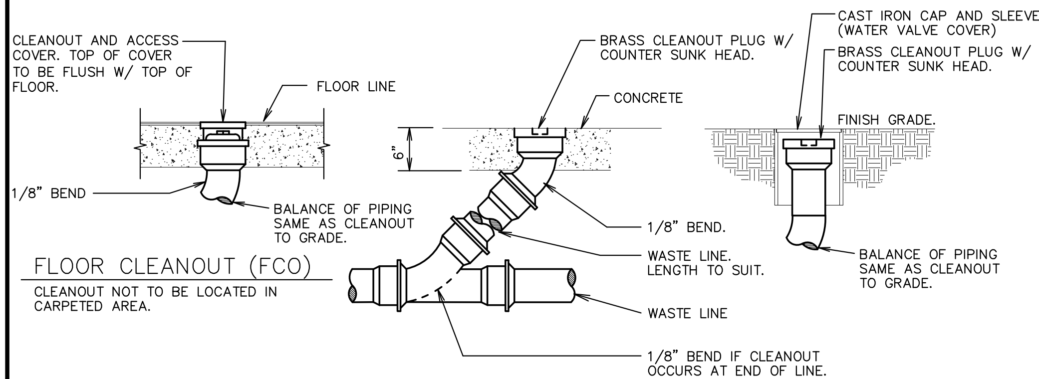
E CLEANOUT DETAILS SCALE: NONE
